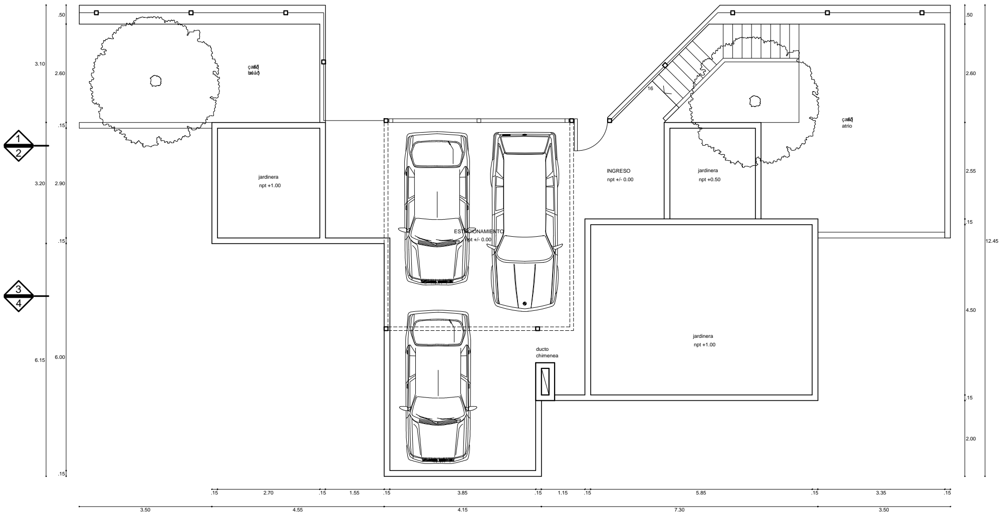
PLANTA NIVEL INGRESO +/- 0.00 - esc: 1/100 -
